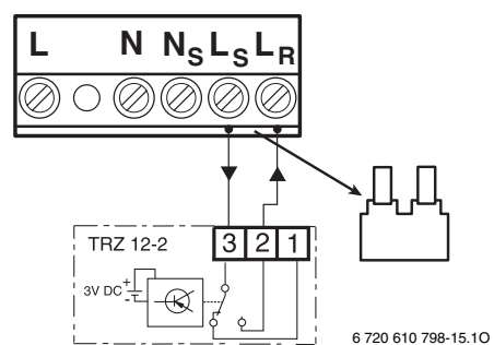
Fig. 17 Collegamento del termostato tipo TRZ .. (230 V AC, eliminare il ponte tra L S e L R )
