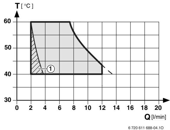
Fig. 26 Diagramma riferito con ingresso a + 15° C
