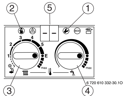
Fig. 30 Elenco degli elementi di comando
