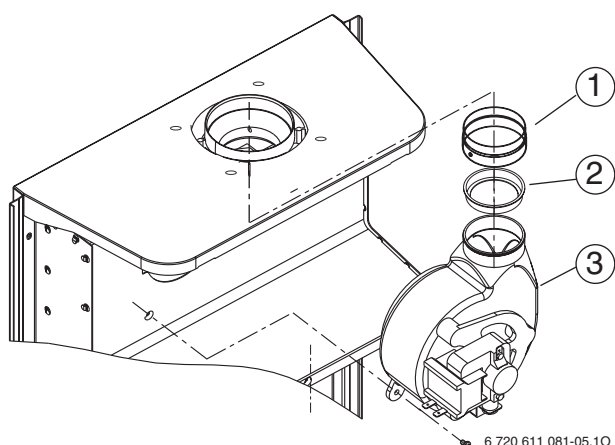
Fig. 10 Smontaggio dell'estrattore
