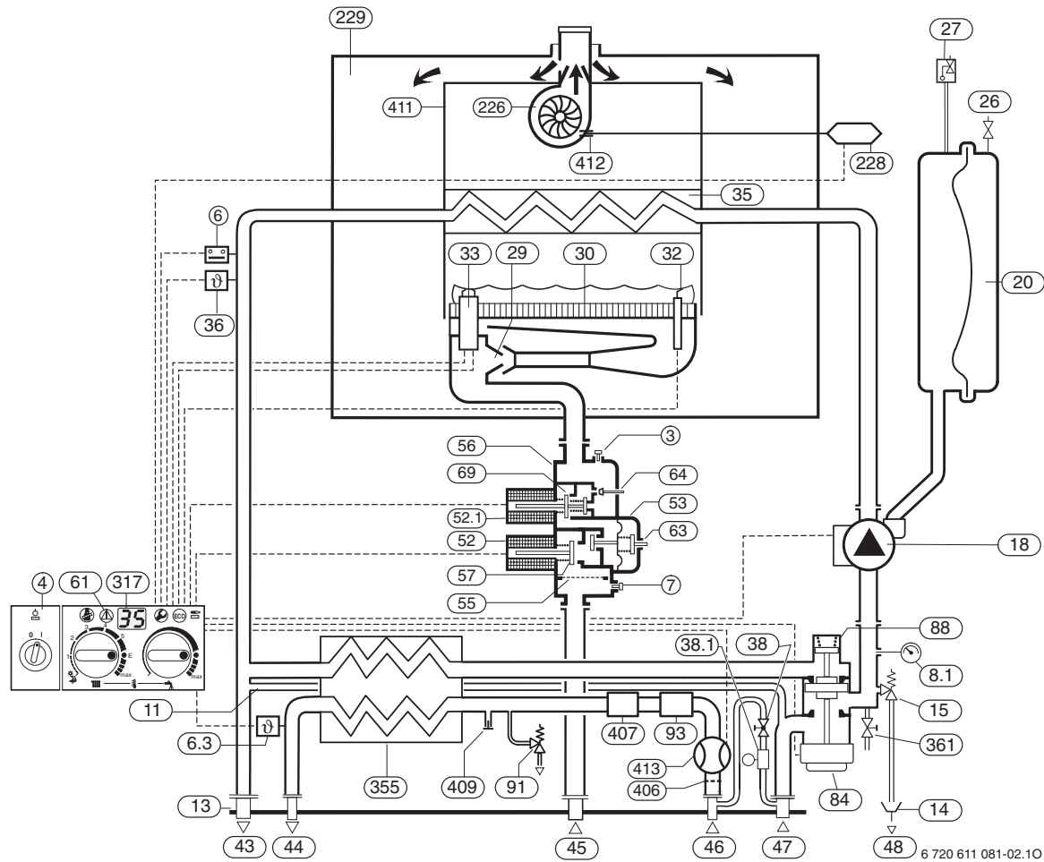
Fig. 2 Schema di funzionamento ZWC
